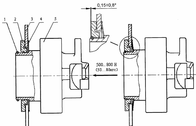
Рисунок 1- Установка интегральной муфты на диафрагменную пружину нажимного комплекта.
