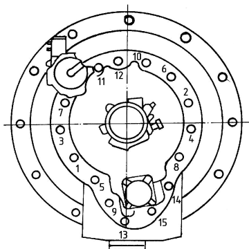
Рисунок 5- Последовательность затяжки гаек крепления картера демультипликатора.
