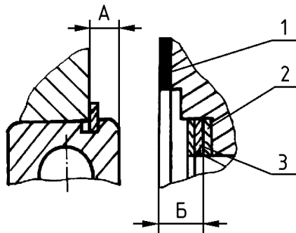
Рисунок 2- Регулировка осевого люфта вторичного вала.
