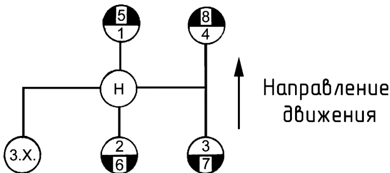
Рисунок 1-Схема положений рычага переключения передач.
